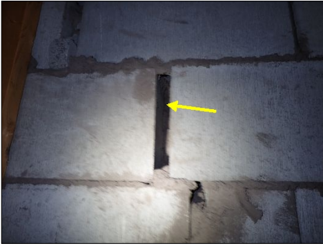
Joint de mortier manquant, par endroits
